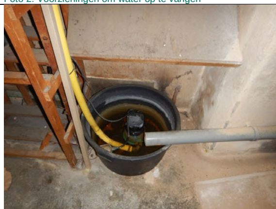
Foto 4: Voorzieningen om water op te vangen en af te voeren
